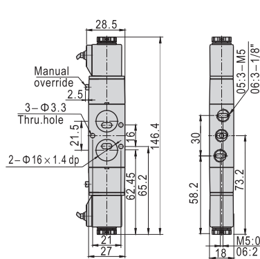
4M120(Grommet)
