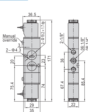
4M220(Grommet)
