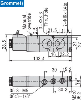
4M120(Grommet)
